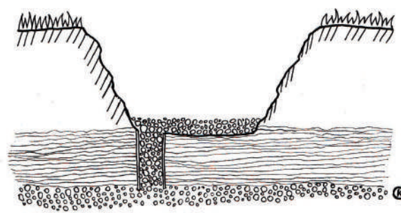
DRENAJE VERTICAL
